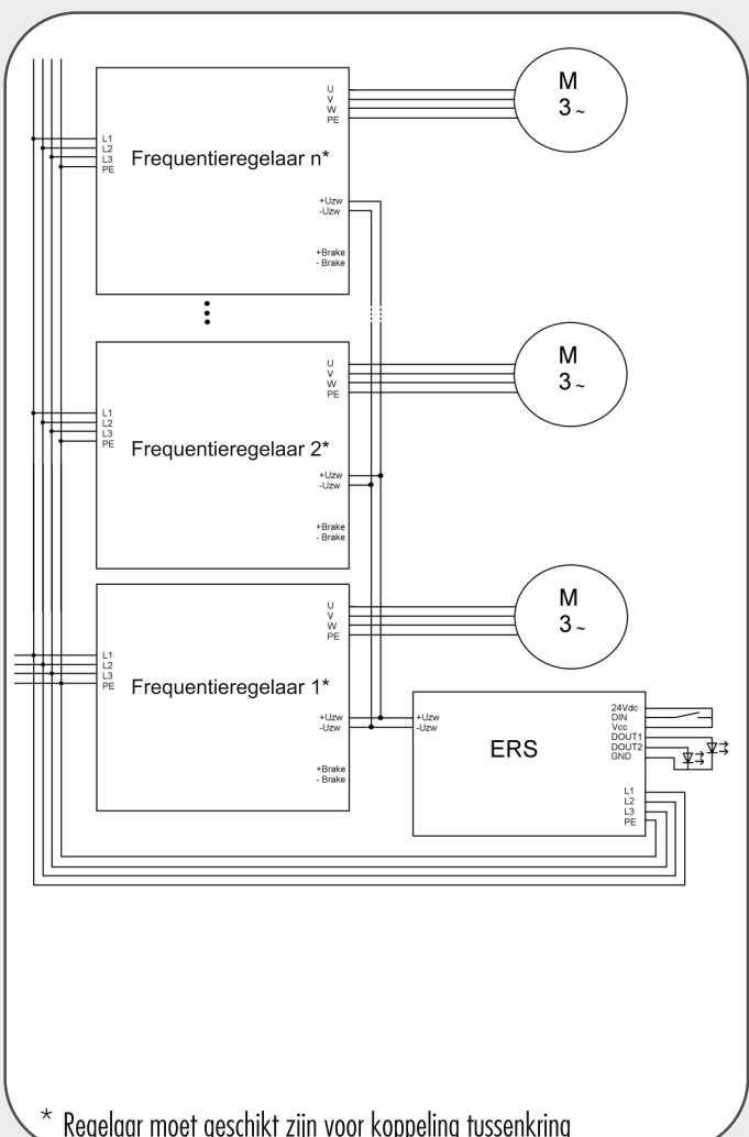
3. Aansluitvoorbeeld tussenkringen gekoppeld met één ERS
