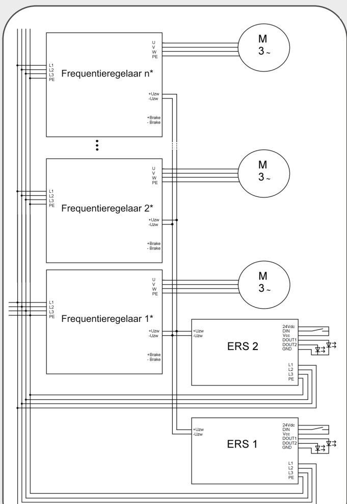
4. Aansluitvoorbeeld tussenkringen gekoppeld met meerdere ERS
