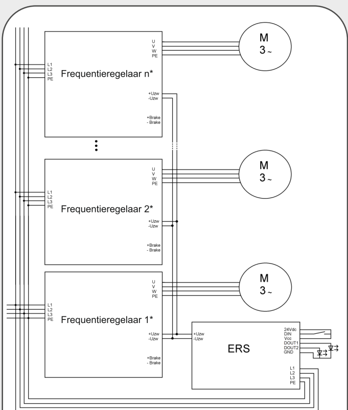
3. Aansluitvoorbeeld tussenkringen gekoppeld met één ERS
