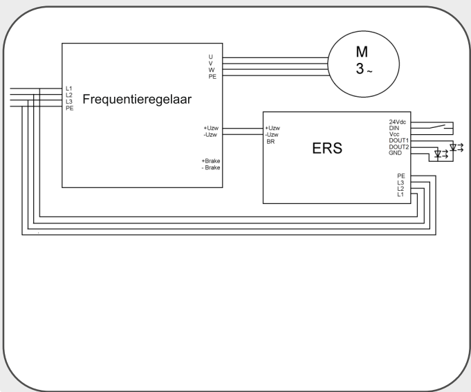
1. Aansluitvoorbeeld frequentieregelaar met ERS
